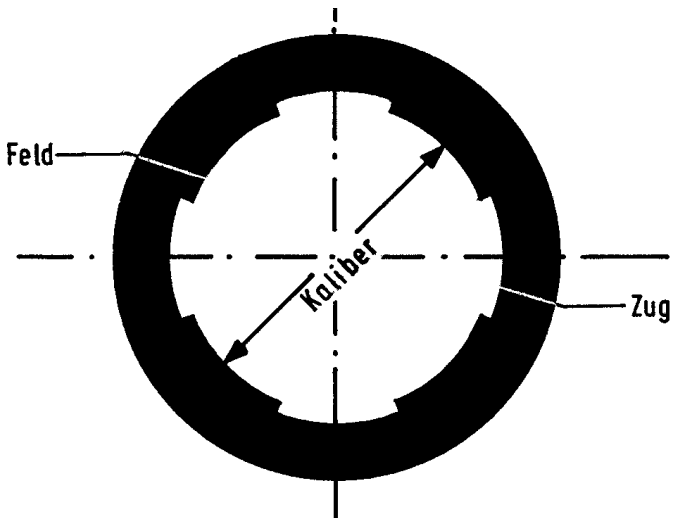
Rohrquerschnitt
