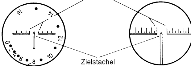
Bild 207 Stricheinteilung
