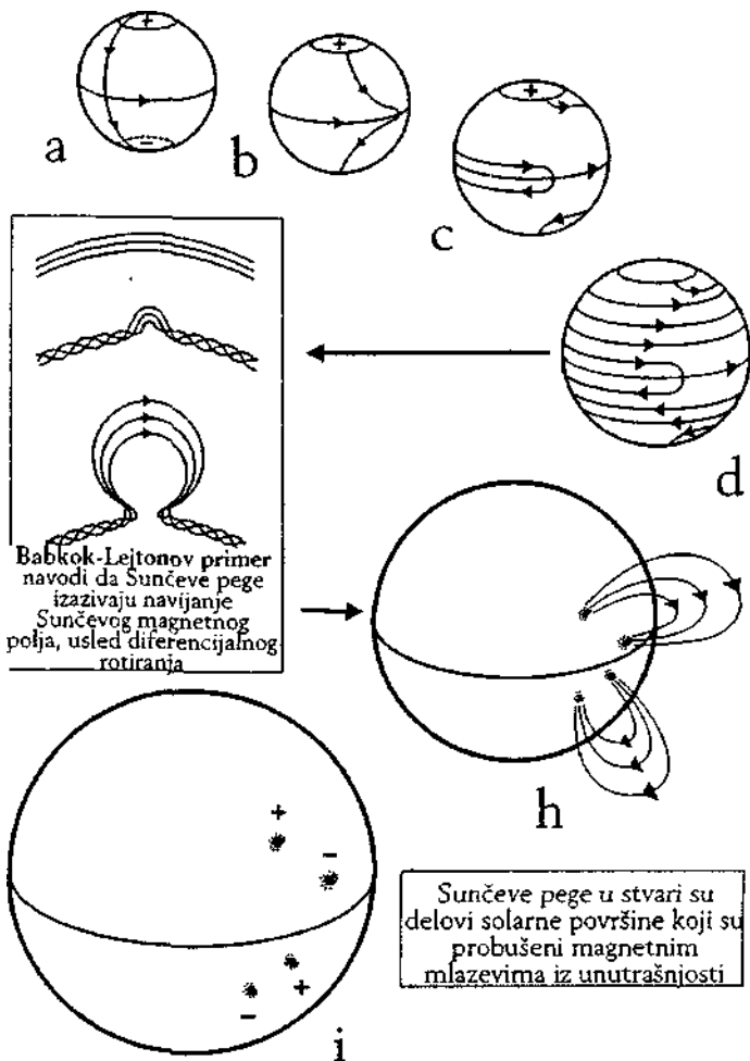
Slika A17: Babkok Lejtonov primer. Prema ovom primeru osnovni mehanizam koji je odgovoran za aktivnost Sun evih pega jeste namotavanje Sun evog magnetnog polja Sun evom diferencijalnom rotacijom.
