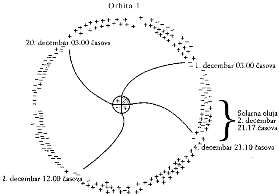
Slika A38: Podeljena struktura solarnog vetra koju je utvrdio Interplanetarni kosmi ki brod br. 1 (IMP), 1963. godine.
