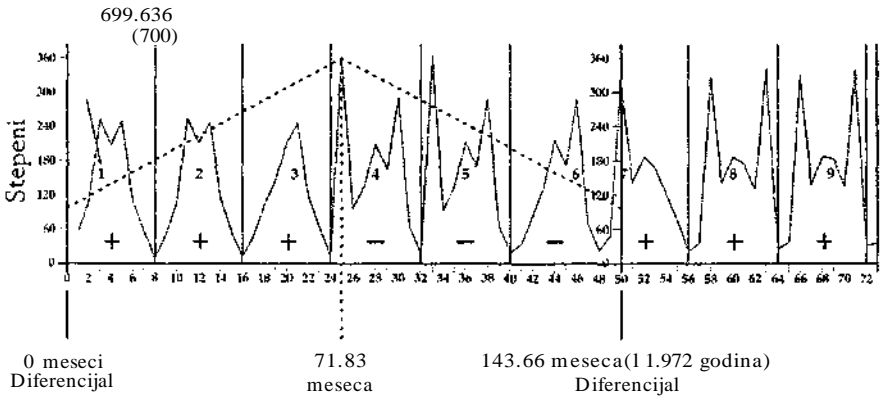
Slika A54: Grafikon analize prvih šest mikrociklusa diferencijalne aktivnosti mikrociklusa Sun evih pega. Kretanje je prikazano isprekidanom linijom i potvr uje jednacinu y = 96.2 + / 1.886153846 x . Dakle, diferencijal potvr uje strmi zup asti oblik krive koji raste i pada svakih 11.97166 godina, predstavljaju i poluciklus diferencijalne aktivnosti. Da bi grafi ki predstavili impulse 4, 5 i 6, potrebno je okrenuti polaritet polja E svaka tri mikrociklusa. Ovo ne može da se postigne u dvodimenzijalnom obliku i objašnjava o igledno vizuelno izvrtanje kod impulsa 4,5i6. Izgleda da negativne vrednosti nisu dozvoljene u ovim jedna inama, navode i da je pravilo kvadrata nerazdvojivo u procesu navijanja. Na primer, +4 na kvadrat iznosi 16, isto kao i -4. Negativne vrednosti u okviru ove šeme mogu da se preokrenu bez menjanja podataka.
