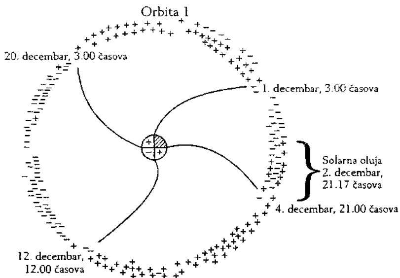
Slika A61: Struktura sektora solarnog vetra koju je utvrdio Interplane tami kosmi ki brod br. 1 (IMP1) 1963. godine, prikazuje solarnu oluju koja traje od 2. do 4. decembra.
