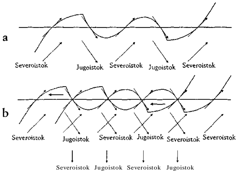
Slika A26. (a) Neutralni omota prikazuje pravac polja. (b) Neutralni omota se pomera u odnosu na osnovni ciklus svakih 187godina. Dakle, bitovi se pomeraju duž 97 ognikrocikli nog niza. Dok se premešteni bitovi sudaraju, Sunceve neutralni omota efektivno menja pravac u pore enju sa inicijalnim pravcem polja, što je ozna eno strelicama.
