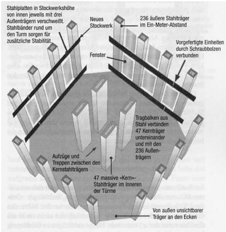
Vereinfachter Turmquerschnitt.
