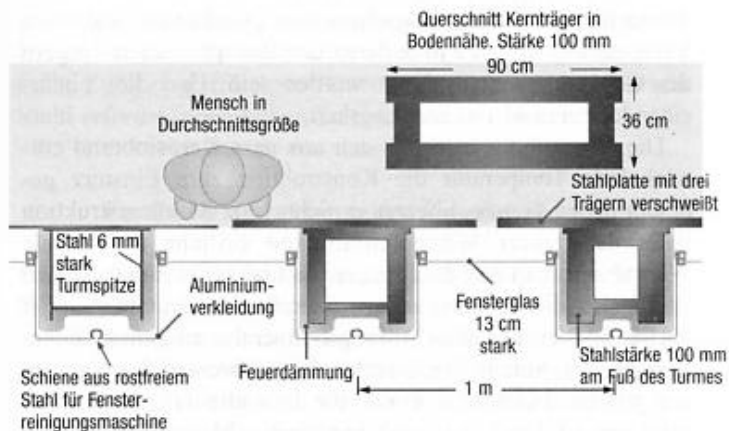
Querschnitt der Außenträger. Die Stahlstärke der drei Säulen ist unterschiedlich, links der Träger in der Nähe der Turmspitze, rechts in Bodennähe. Zum Vergleich: Querschnitt eines Kernstahlträgers in Bodennähe.
