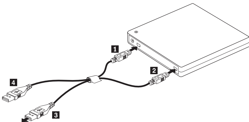
Obrázek 1-2. Konfigurace 2: napájení ze standardní sběrnice USB
