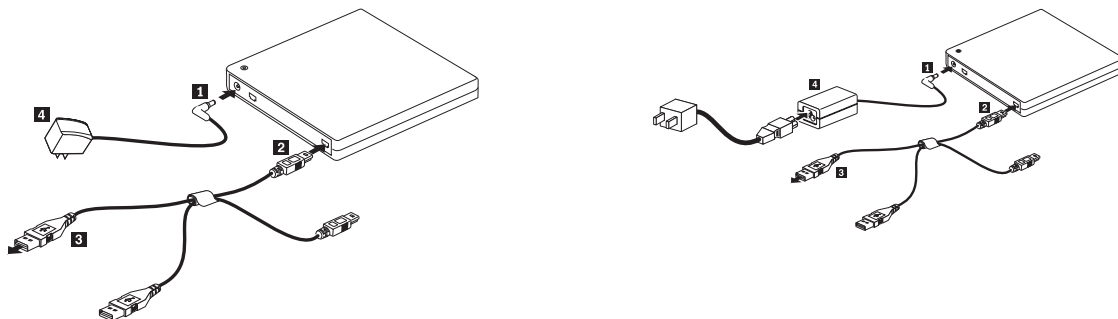
Obrázek 1-1. Konfigurace 1: vlastní napájení (napájecí zdroj)
