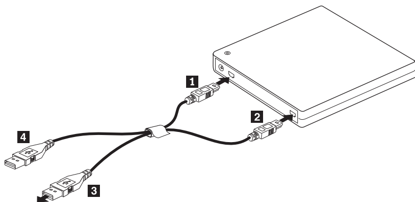
Obrázok 1-2. Konfigurácia 2: Konfigurácia s napájaním z USB
