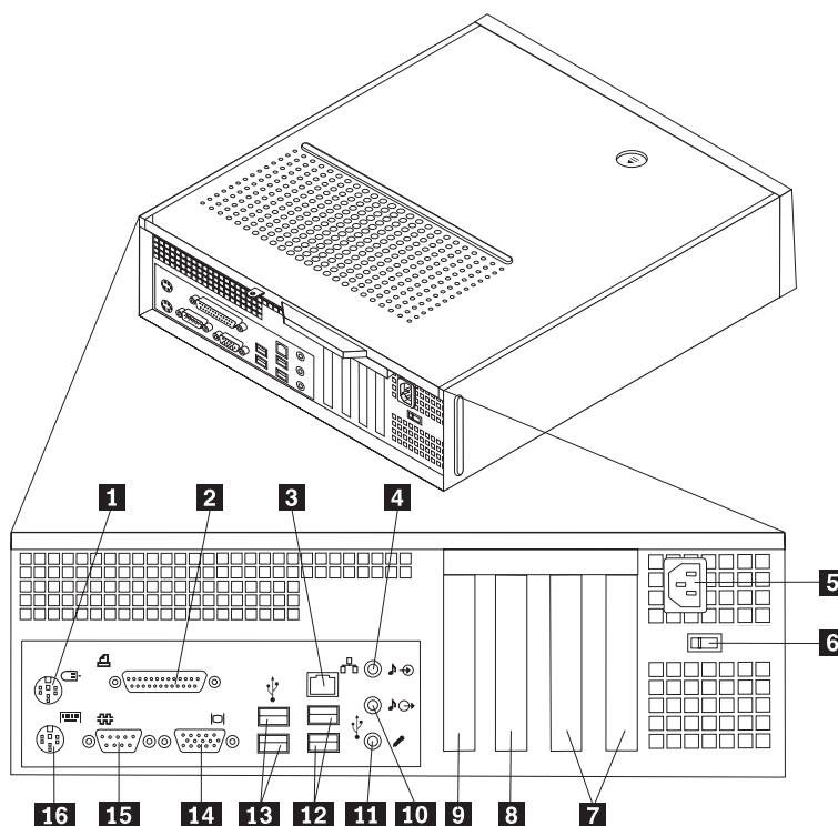
Рисунок 2. Расположение разъемов
