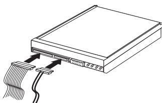
Рисунок 17. Подключение последовательного диска ATA
