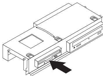
Рисунок 26. Установка нового дисковода для дискет
