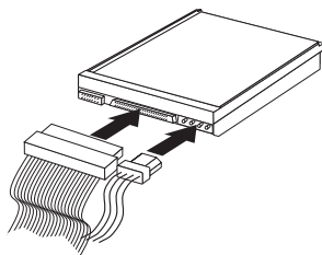
Рисунок 16. Подключение параллельного жесткого диска ATA
