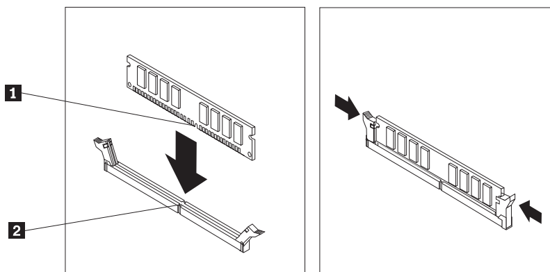
Рисунок 34. Установка модуля памяти
