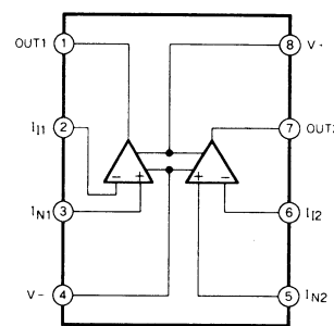
IC3 μPC358G2
