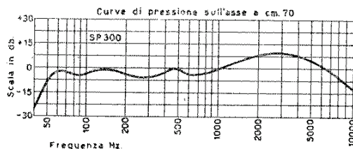
Fig. 2 - Curva di risposta.
