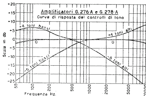
Fig. 4 - Risposta a controlli di tono.
