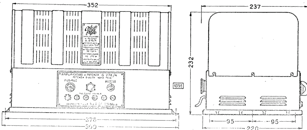
Fig. 11 - Le dimensioni di ingombro dell'unità di potenza G. 278/A. Sulla targhetta frontale, oltre all'interruttore, al fusibile ed alla gemma-sonia, sono chiaramente visibili le indicazioni per la dislocazione delle valvole.
