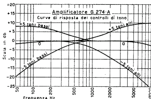
Fig. 4 - Risposta e controlli di tono.
