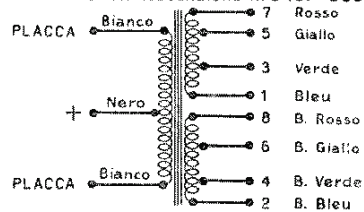
TRASFORMATORE di MODULAZIONE N. 5407-6055
