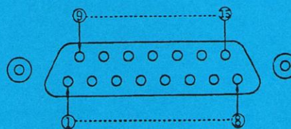
Figura 4.8 - Piedinatura del connettore per amplificatore lineare (vista dall'esterno del pannello posteriore)
