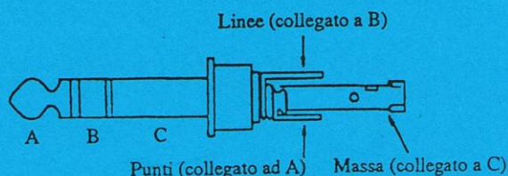
Figura 6.13 - Collegamento di un tasto CW
