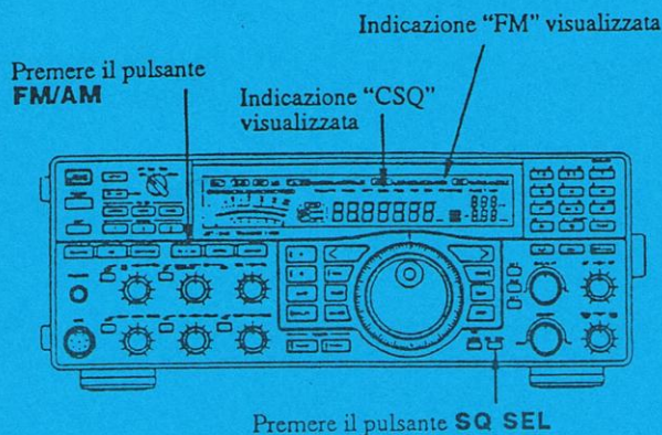
Figura 6.11 - Uso del code squelch
