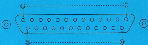
Figura 4.9 - Piedinatura del connettore per app. periferiche (vista dall'esterno del pannello posteriore)
