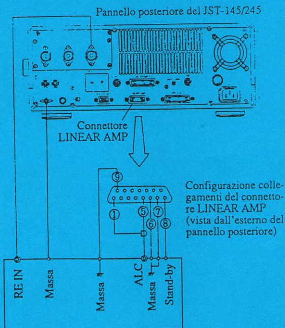
Figura 6.14 - Collegamento di un amplificatore lineare
