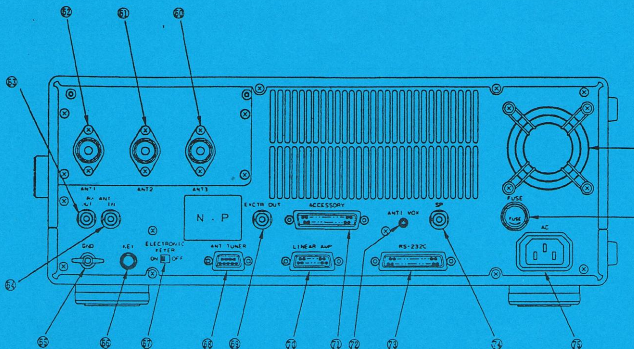
Figura 4.3 - Il pannello posteriore
