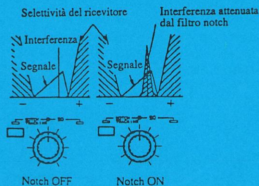
Figura 6.3 - Intervento del filtro notch
