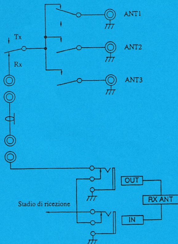
Figura 4.6 - Collegamenti interni degli ingressi antenne
