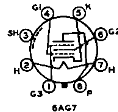
6AG7
