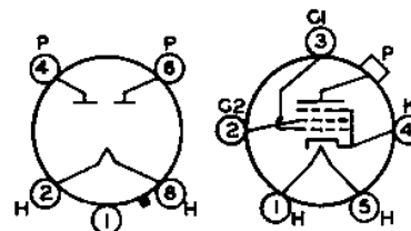
6U4G
