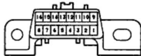
D24 Data Link Connector 3
