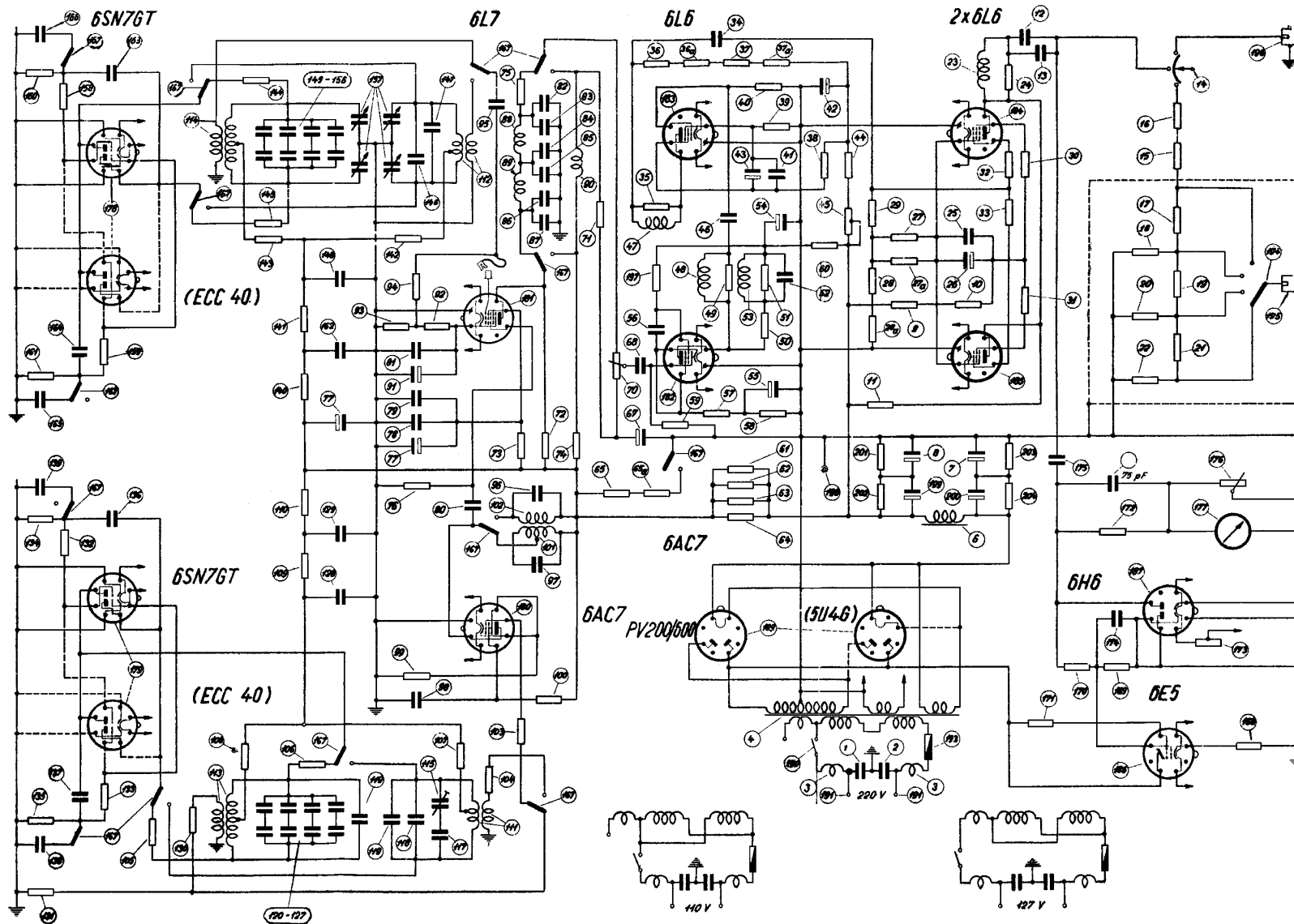
542. 65. ábra. Az EMG 1131 típusú széles frekvenciasávú áramforrás elvi kapcsolási rajza
