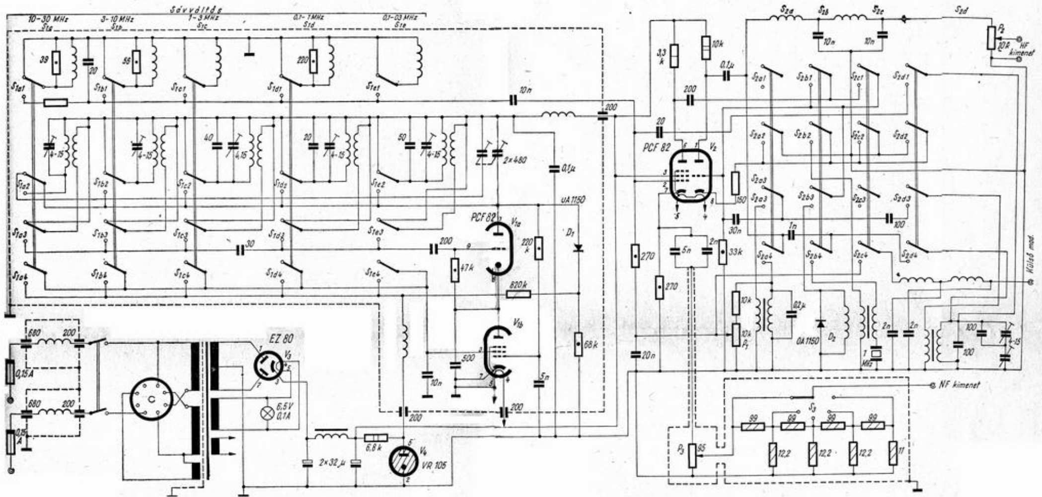
EMG 1166/B típusú üzemi szignálgenerátor kapcsolási rajza
