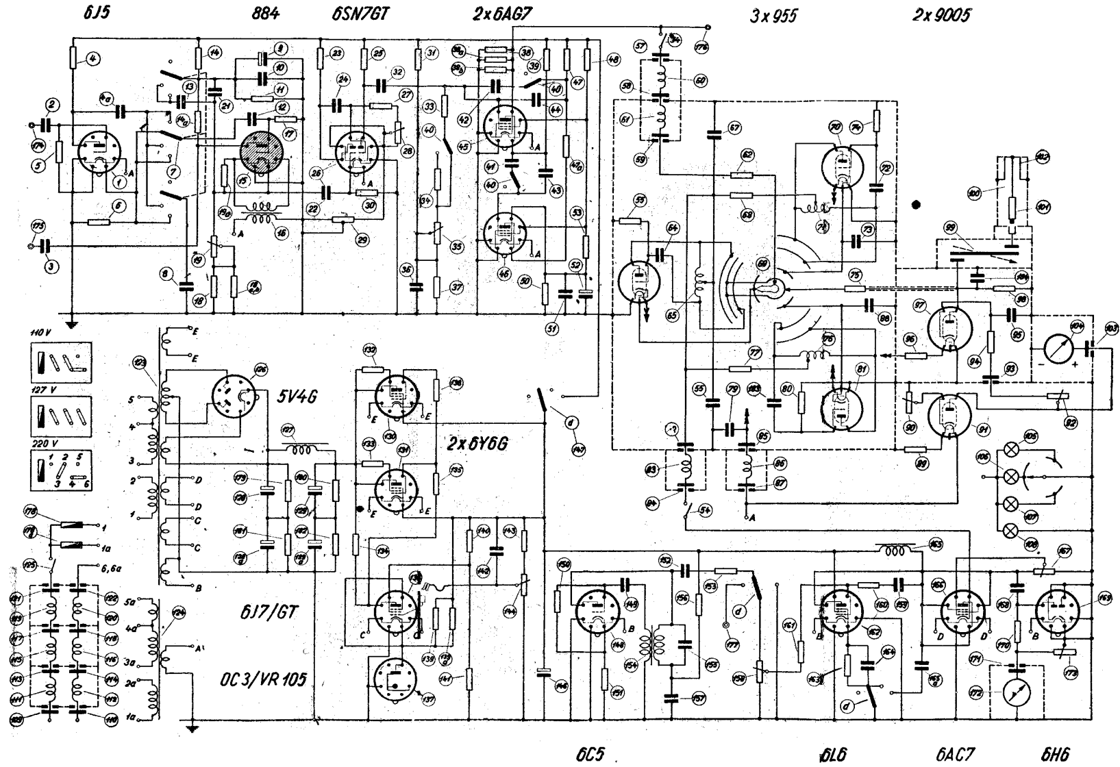
543. 77. ábra. Az EMG 1174 típusú URH rádiófrekvenciás áramforrás teljes kapcsolási rajza
