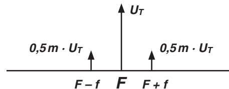
Abb. 1: Spektrumsamplituden und -frequenzen bei AM ( m = 50\% )
