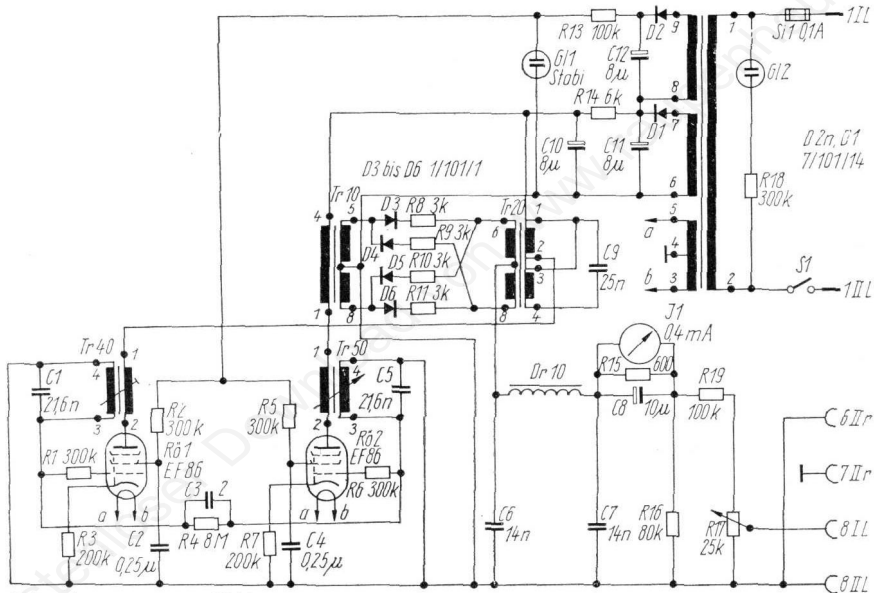
Schwingungssummer GF 1
