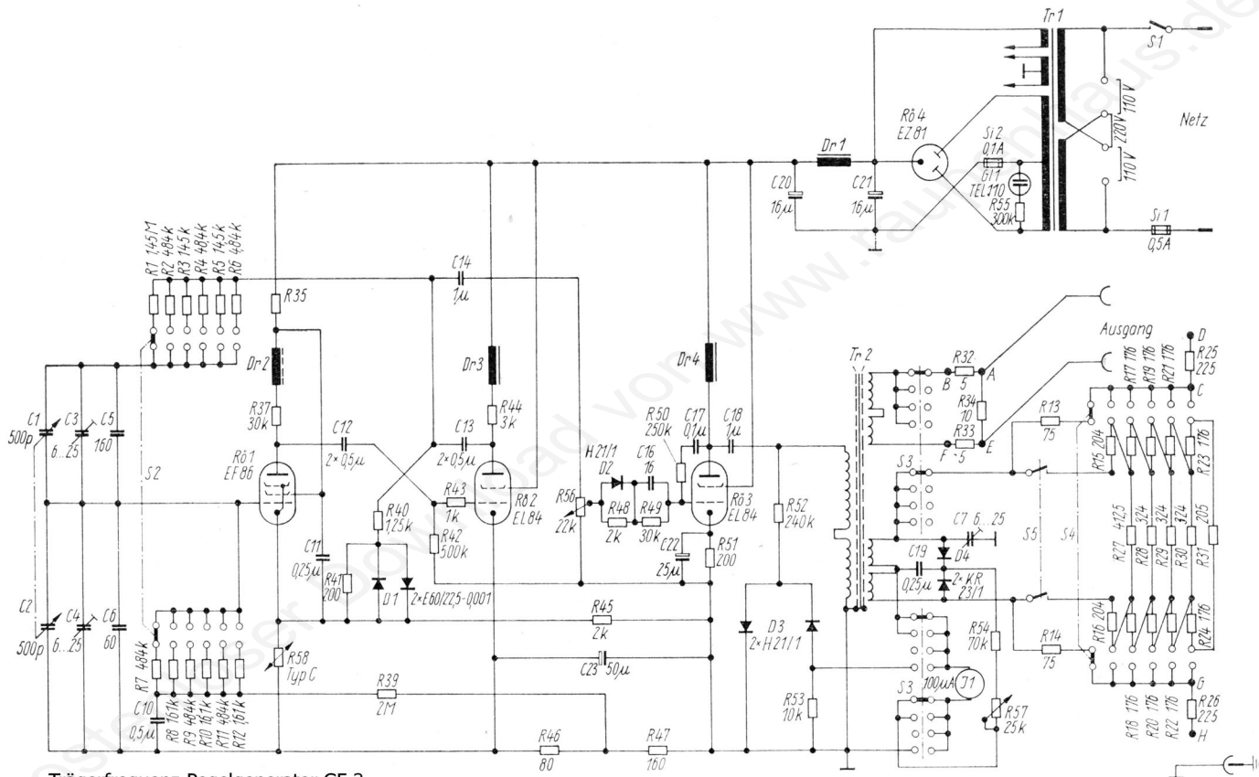
Trägerfrequenz-Pegelgenerator GF 3
