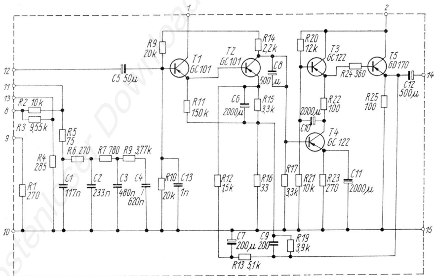
Rauschgenerator NRG 201 - Be 3
