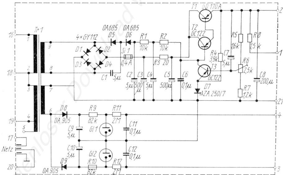
Rauschgenerator NRG 201 - Be 5
