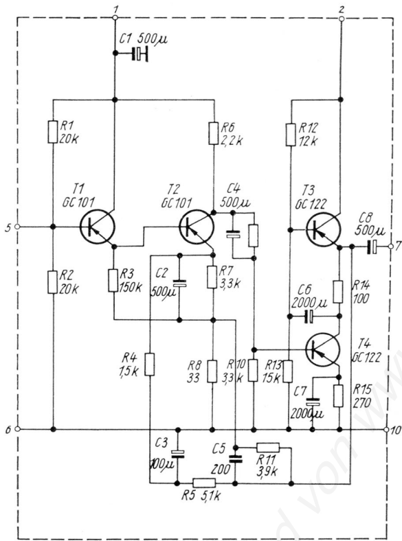
Rauschgenerator NRG 201 Be 2
