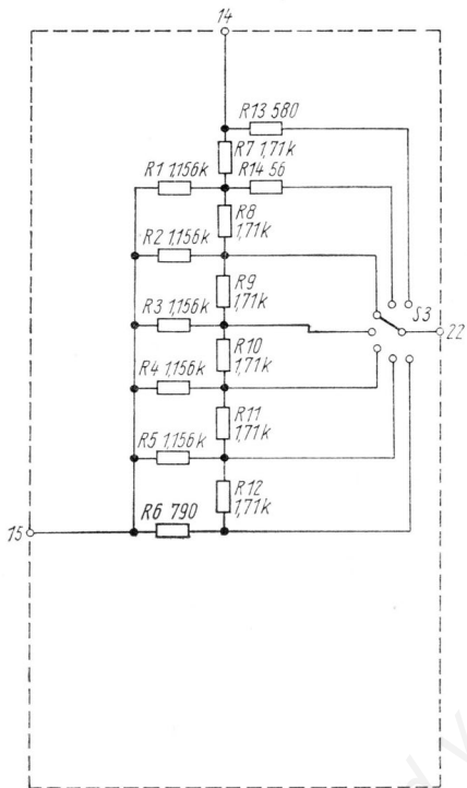
Rauschgenerator NRG 201 Be 4
