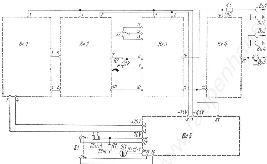
Rauschgenerator NRG 201 - Übersicht
