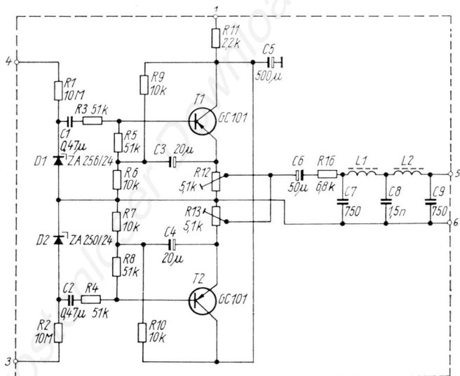
Rauschgenerator NRG 201 Be 1
