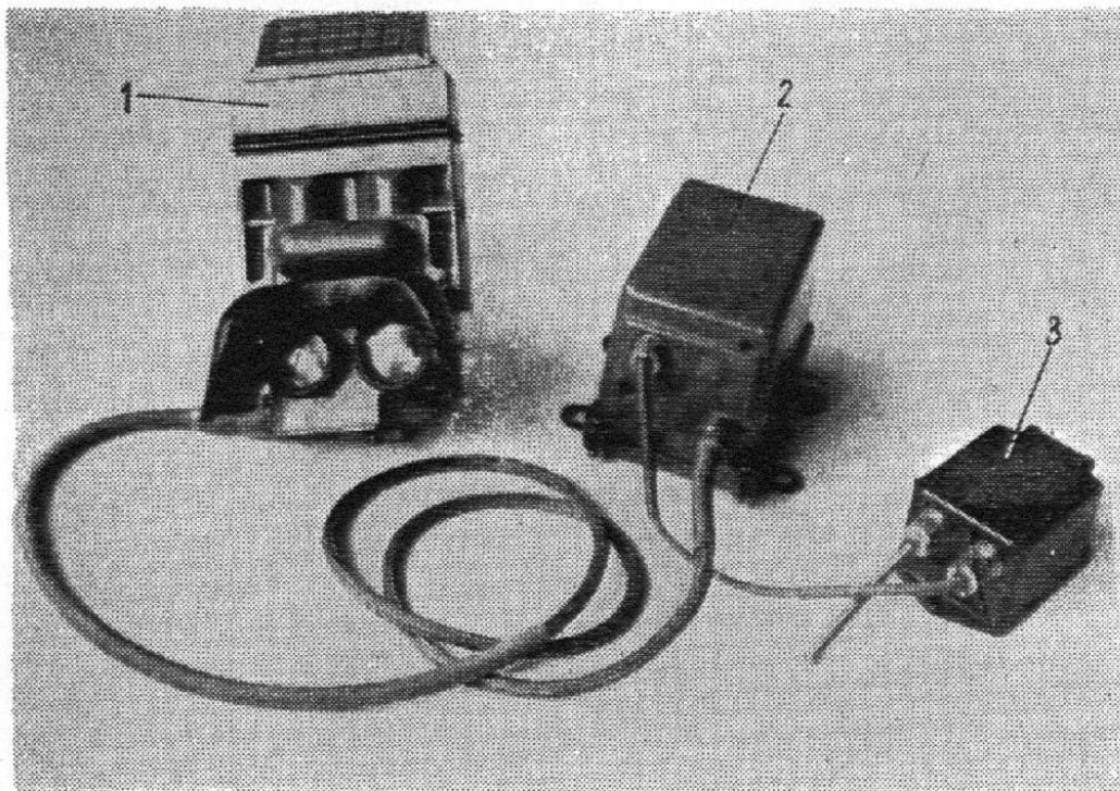
Rys. 63. Noktowizor czołgowy TWN-2 (bez reflektora): 1 — peryskop; 2 — zasilacz; 3 — filtr przeciwzakłóceńowy
