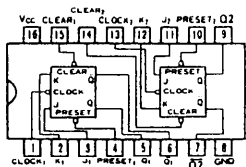
SN74LS112N
