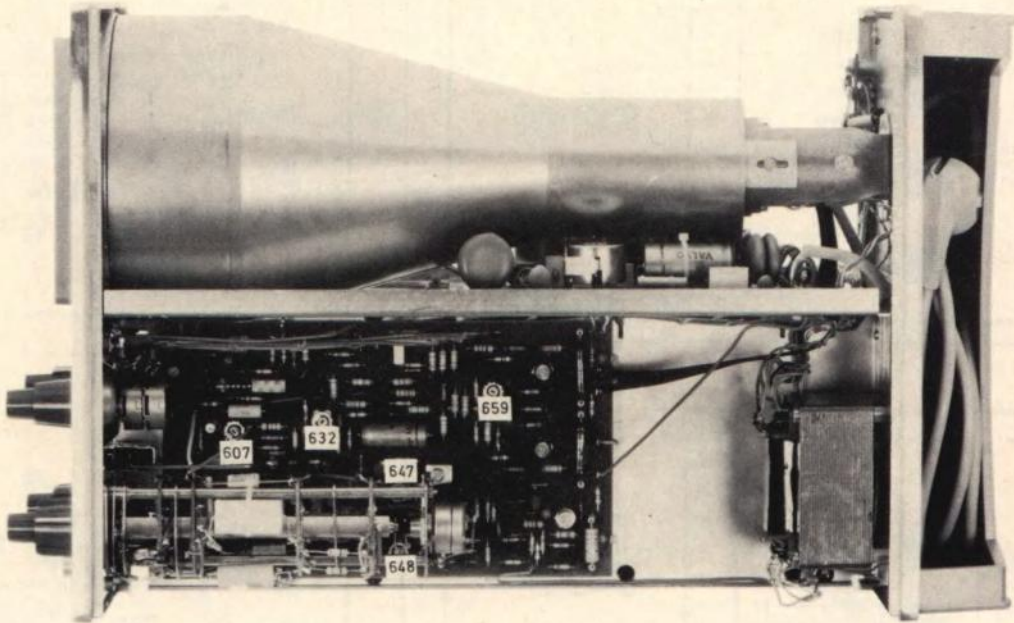
Fig. 10 Abgleichelemente auf UNIT 3
