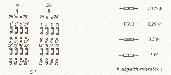
Wirksaltplan E0174/A ab Gerätenummer 72 1201
