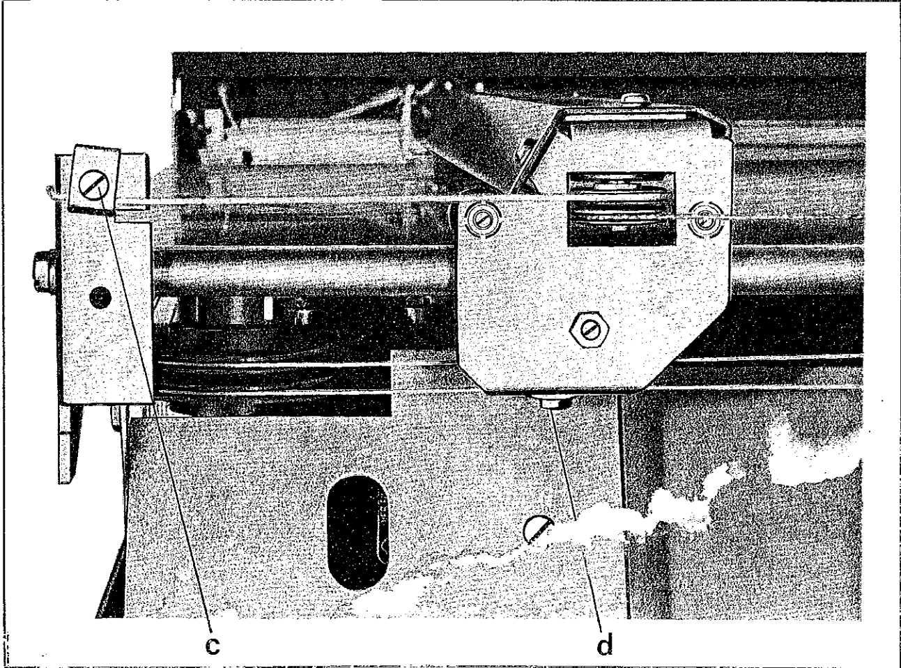
Spannen des y-Seiles und Ausrichten des x-Schlittens
